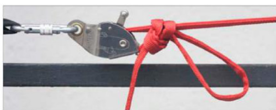
Nudo de pescador para bloquear el anclaje
